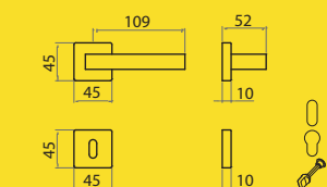
1 Ros 45x45 Mont. n°50-51
