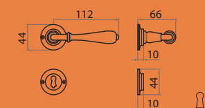
3 Ros 45x10 V.V. Mont. n°107
