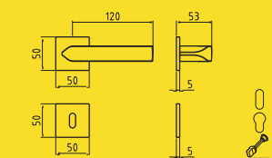
1 Ros 50x50x5 (molla ambidestra - maniglia non solidale)
