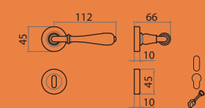
1 Ros 45X9 Mont. n°88-89
