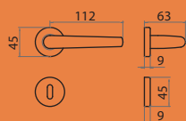
3 Ros 45X9 Mont. n°88-89
