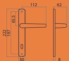
2 Placca STRETTA Mont. n°37
