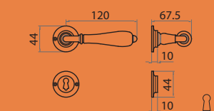
3 Ros 45x10 V.V.
