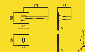
1 Ros 50x50x5 (molla dx e sx - maniglia non solidale)
